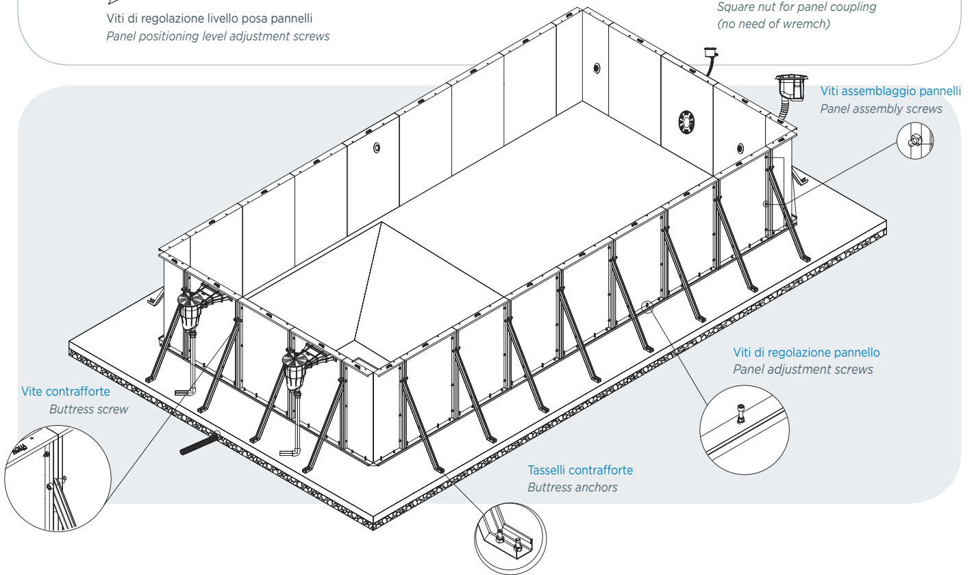
Sistema a incastrò senza saldature Snap-on system without welds
