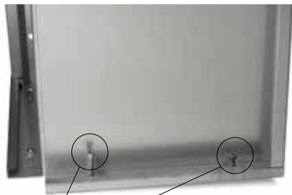
Viti di regolazione livello posa pannelli Panel positioning level adjustment screws
